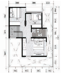
1 DENAH LANTAI ATAS SKALA 1:100
